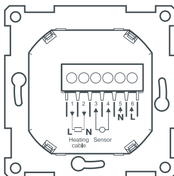
Рис. 2 Соединения термостата
