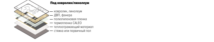
Рис. Схема монтажа теплого пола CALEO под ковролин или линолеум
