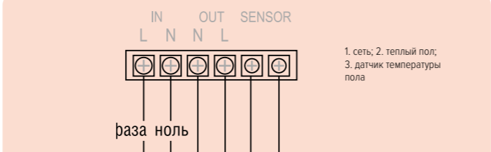
Рис. Схема монтажа теплого пола CALEO под ламинат или паркетную доску
