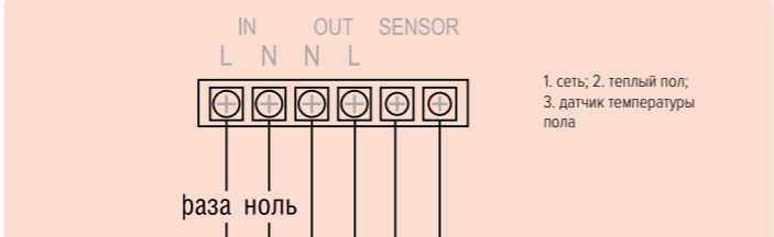
Рис. Схема монтажа теплого пола CALEO под ламинат или паркетную доску
