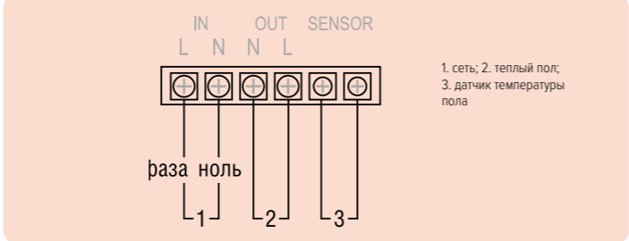
Рис. Схема монтажа теплого пола CALEO под ламинат или паркетную доску
