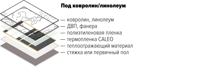
Рис. Схема монтажа теплого пола CALEO под ламинат, ковролин, линолеум
