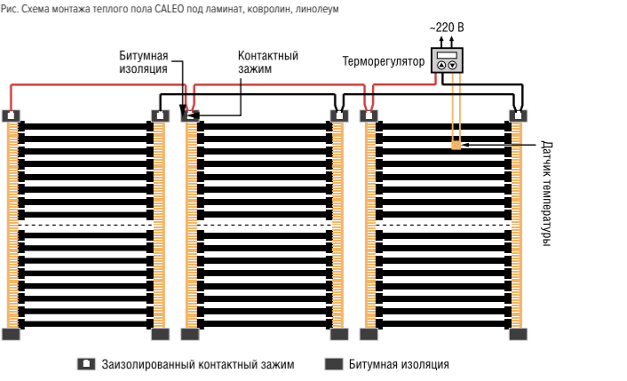
Рис. Общая схема подключения термоплёнки CALEO
